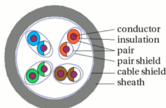
Gambar 3.50 S/STP
