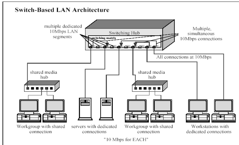
Gambar 3.37 Cara kerja Switch
