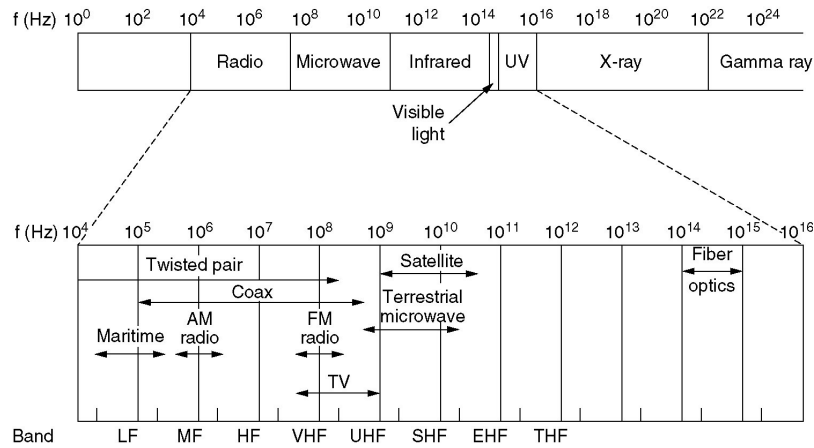
Gambar 3.55 Spektrum Elektromagnetik
