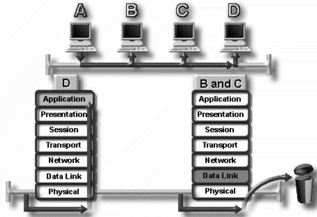
Gambar 2.18 CSMA/CD
