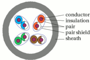
Gambar 3.49 STP
