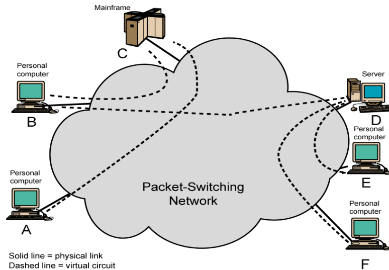
Gambar 3.45 Penggunaan X.25
