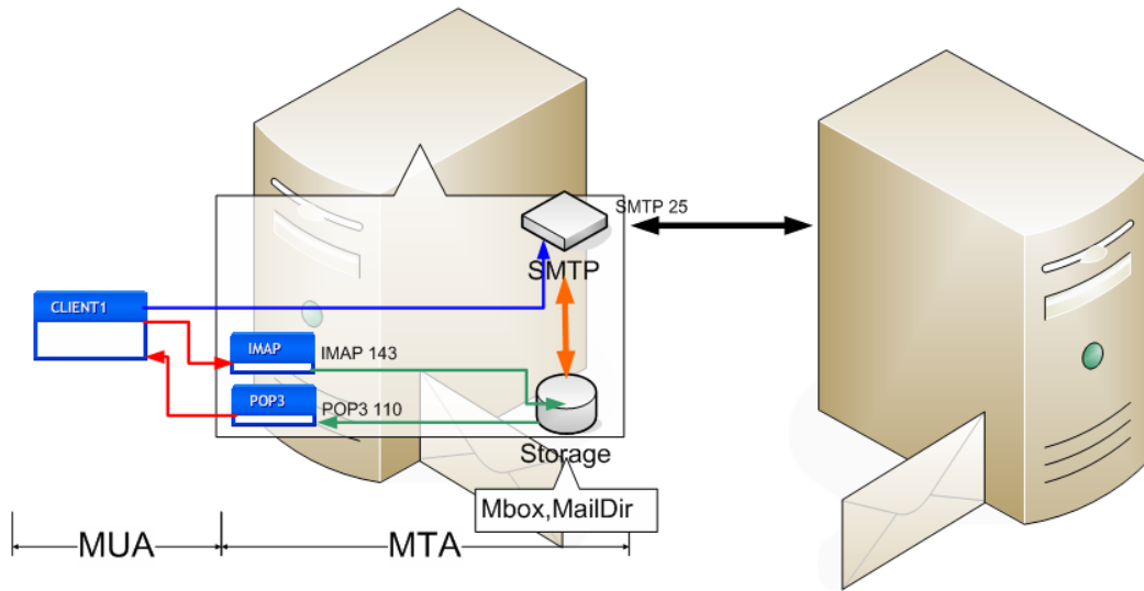
Gambar 12.104 Cara kerja EMAIL
