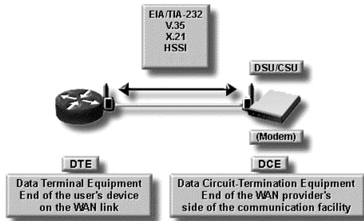
Gambar 3.42 Bentuk sambungan fisik perangkat WAN
